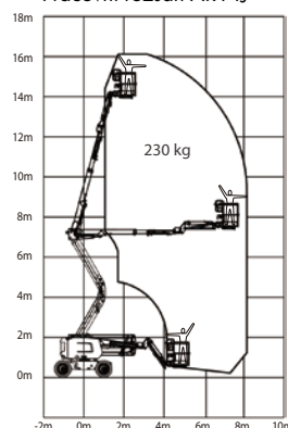
Pracovní rozsah AR14J
