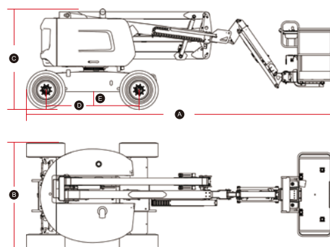
Pracovní rozsah AR14J
